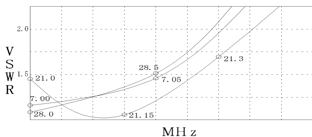
VSWR特性
