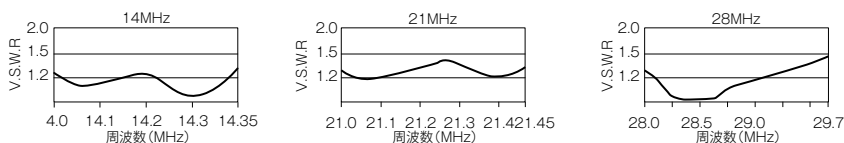
T3-11DX V.S.W.R.特性表
