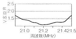
HX-330 V.S.W.R.特性表
