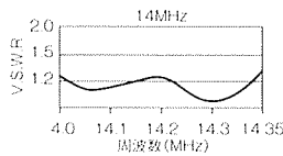
T3-11DX V.S.W.R.特性表
