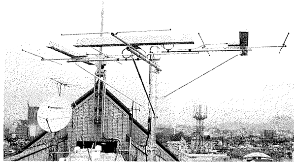
コミュニティFM 防雪型3素子3方向設置
